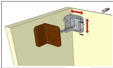
Крепление подвески к боковой стенке шкафа
