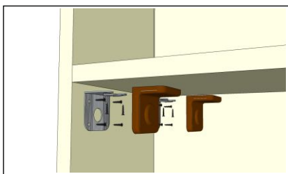
Наличие дополнительных отверстий позволяет использовать подвеску как крепежный уголок
