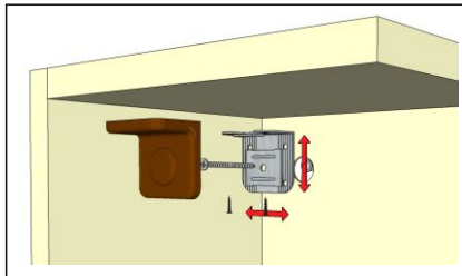
Крепление подвески к крышке шкафа
